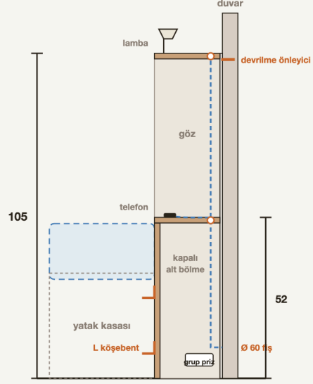
Başlık kesiti
